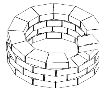
Figure 4. Layer 4 / Cap layer
